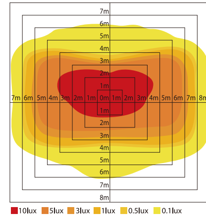
床照度分布図 高さ:3m 白色タイプ
